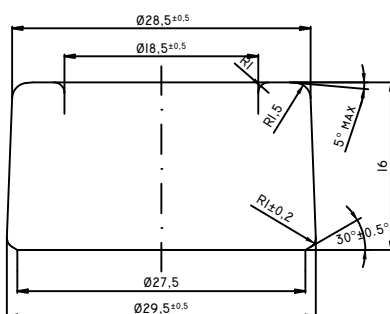
PARTICOLARE IMBOCCATURA SCALA 3:1
